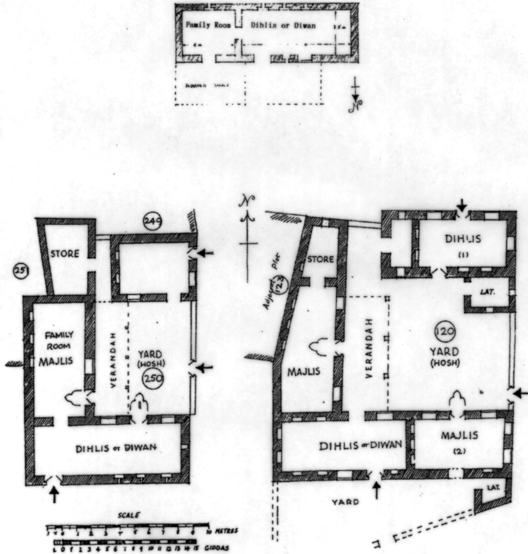
الشكل ٤: مسقط أفقي للمنازل في سواكن - النوع الأول. (نقلًا عن: Greenlaw 1976).
